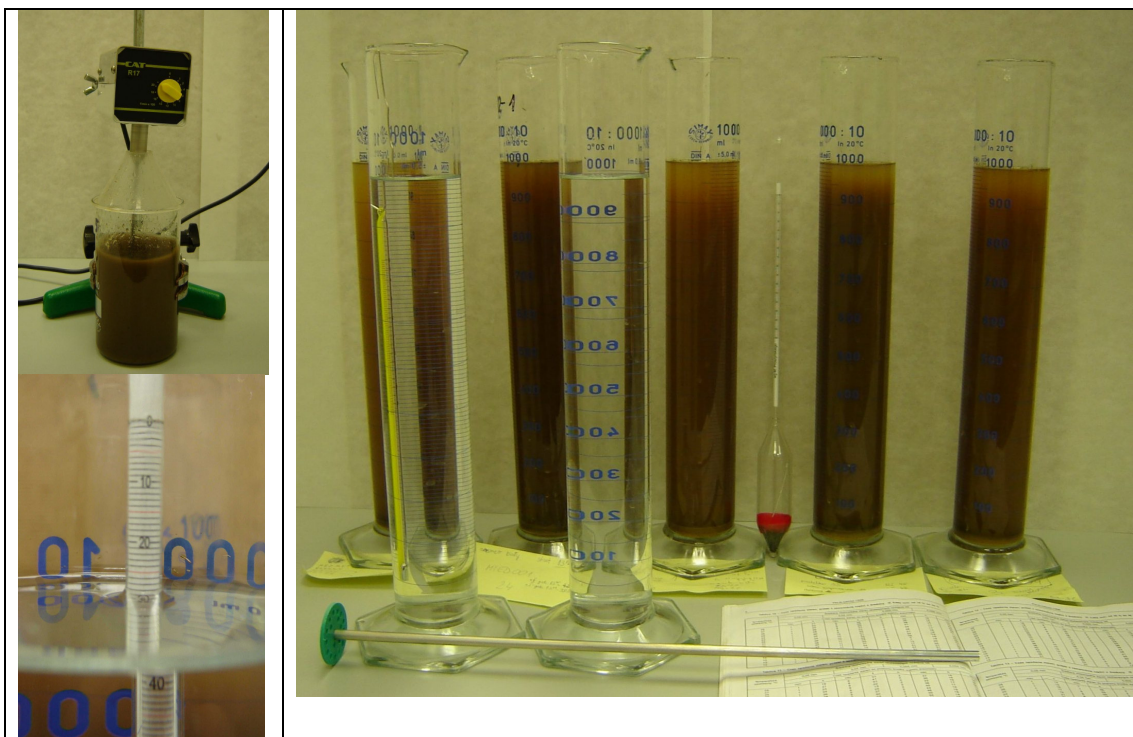
Rys. 4. Sprzęt stosowany w metodzie areometrycznej
