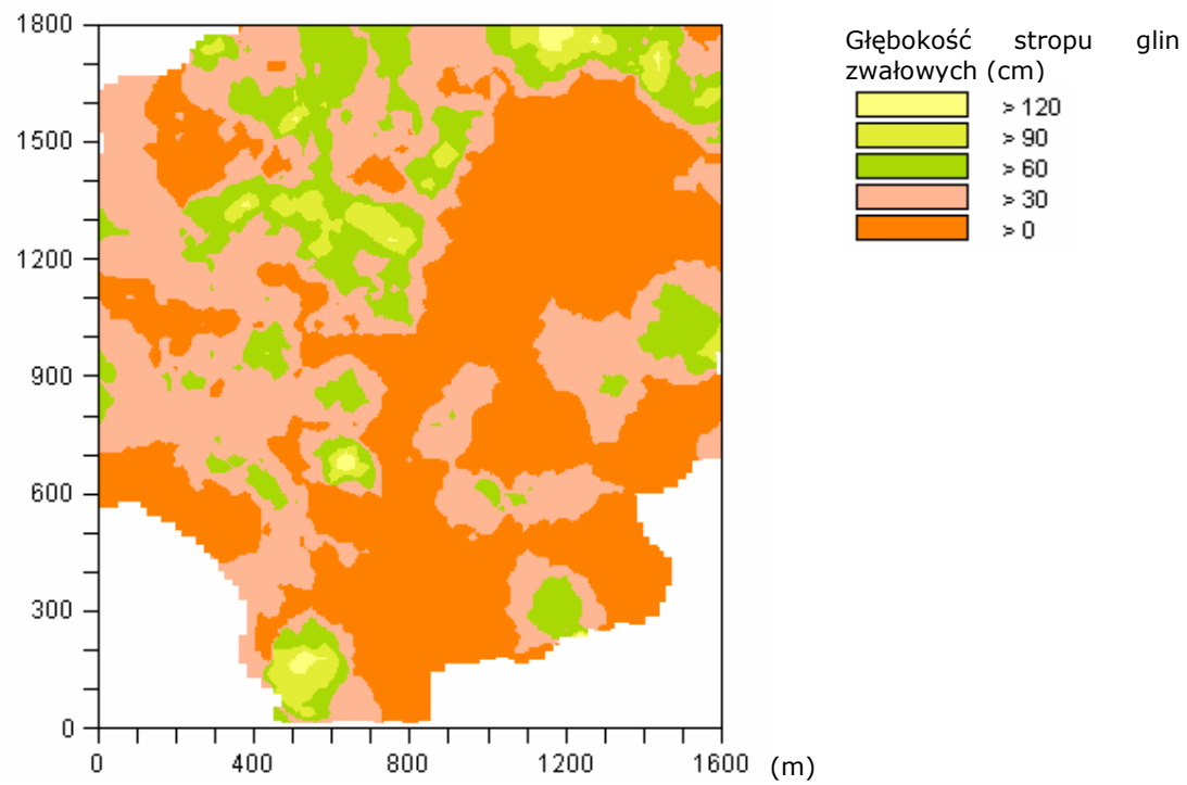
Rys. 7. Przykład przestrzennego zróżnicowania miąższości utworów piaszczystych w obrębie falistej moreny dennej, Przybroda k/ Poznania (odległości w metrach).
