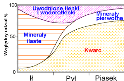
Rys. 2 Schemat składu mineralogicznego frakcji granulometrycznych według Brady i Weil (1999)
