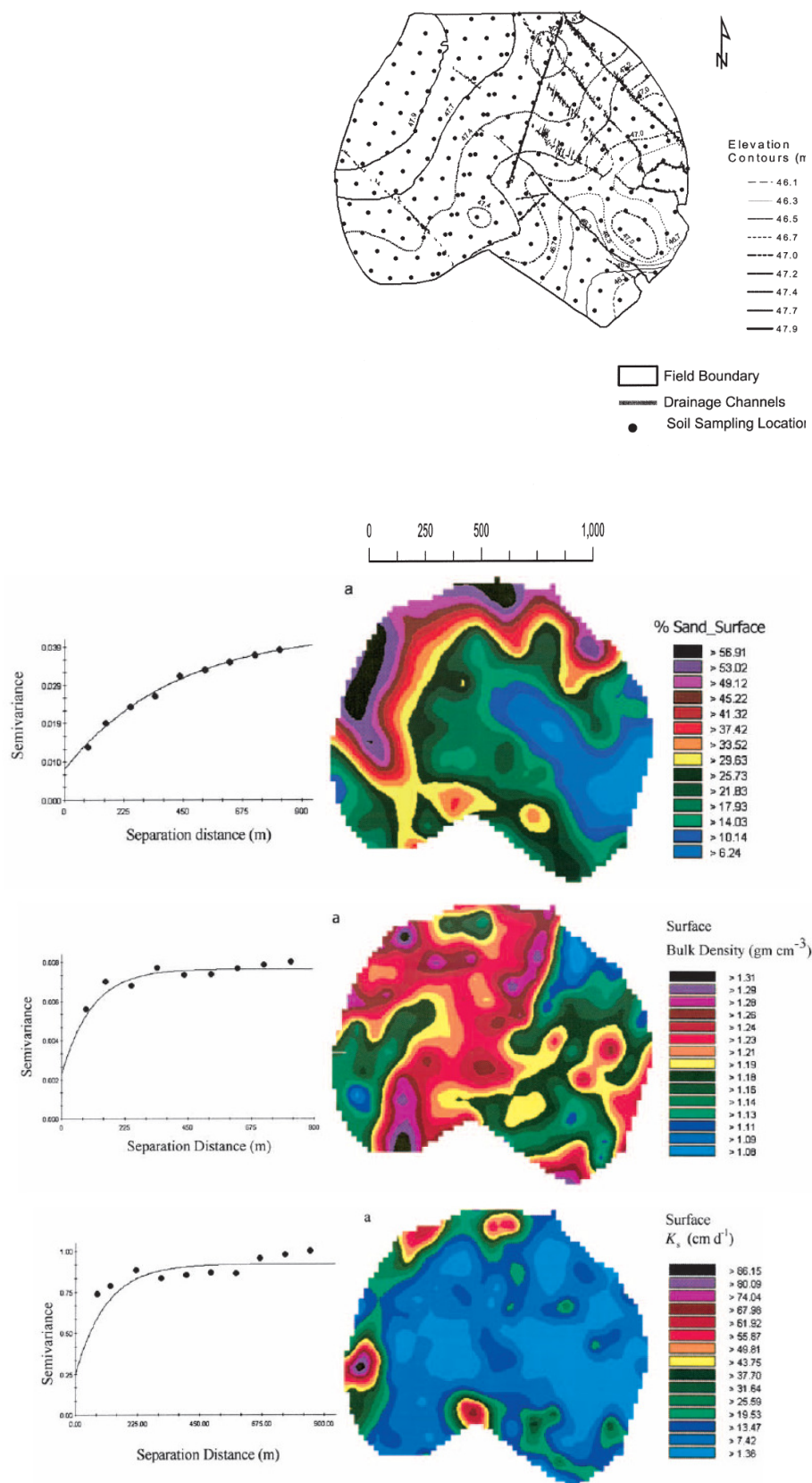
Rys. 8. Przykład zróżnicowania w skali pola zawartości frakcji piasku, gęstości objętościowej i współczynnika filtracji (Igbal i in. 2005; SSSAJ vol. 65).
