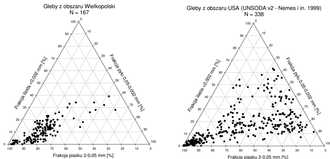
Rys. 6. Porównanie uziarnienia gleb z obszary wielkopolski i USA
